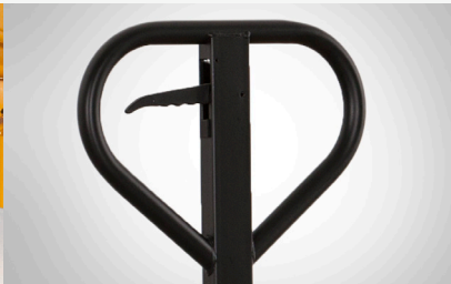
Poignée en forme de goutte d'eau munie d'un levier à 3 positions pour le contrôle de la charge
