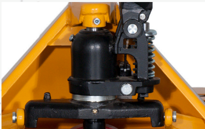
Pompe hydraulique avec soupape de dérivation en cas de surcharge
